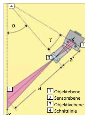
Bild 5: Optikschemata einer Scheimpflug-Anordnung
